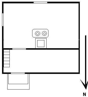
Stuorommet planskisse 1. etg ca 1925
